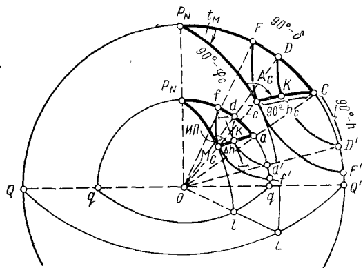
Рис. 89. Обоснование метода расчета элементов высотной линии положения
