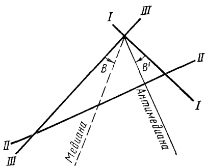
Рис. 107. Построение антимедианы
