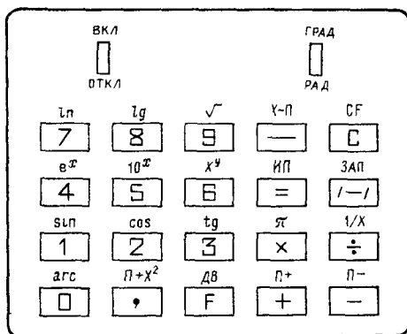
Рис. 80. Клавиатура ЭКВМ
