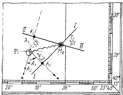
Рис. 93. Пример прокладки линий положения на меркаторской карте
