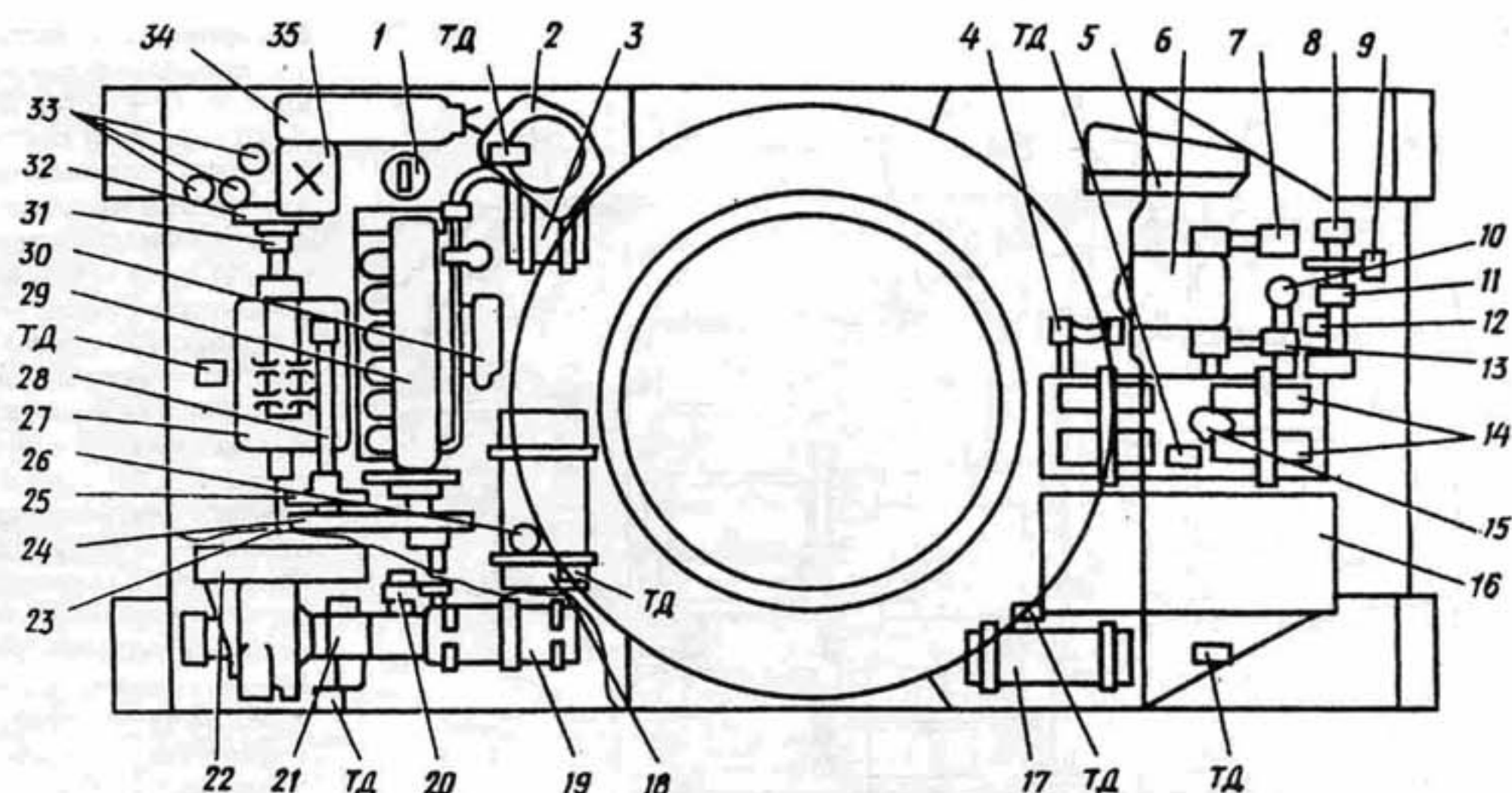
Схема размещения узлов и агрегатов в корпусе ГМ-575:
