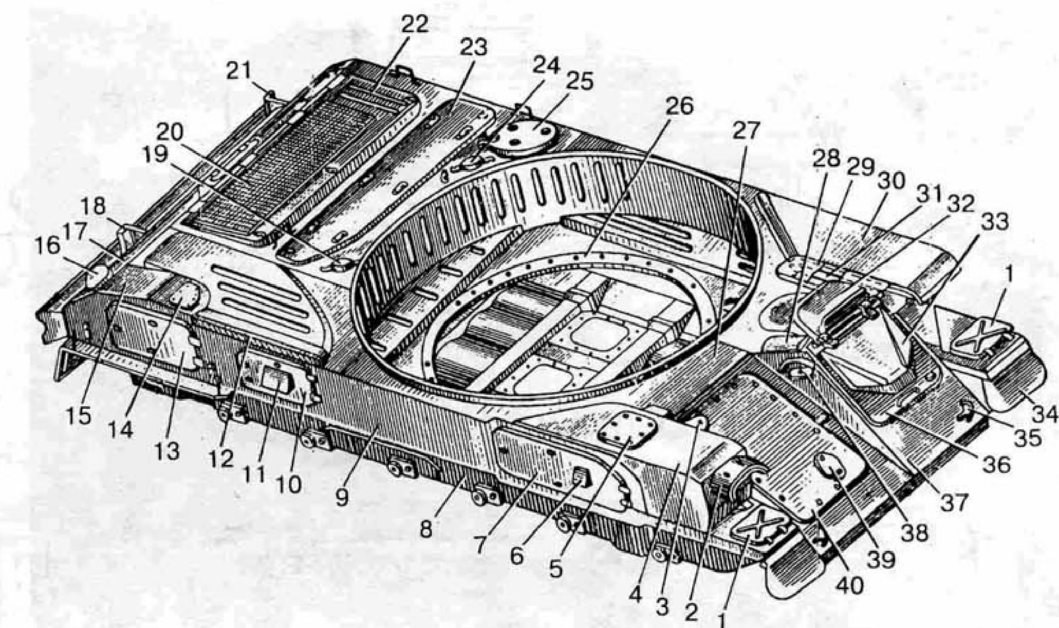
Корпус ЗСУ-23-4:
