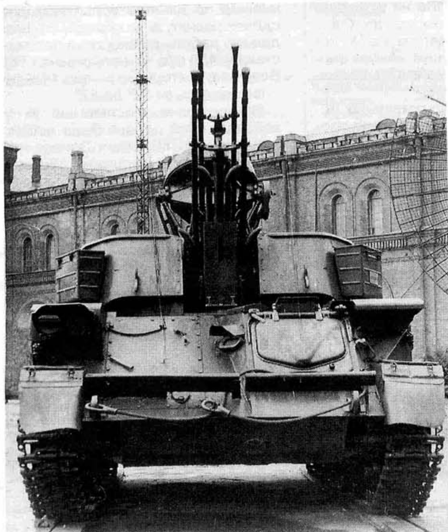
ЗСУ-23-4В в экспозиции Военно-исторического музея артиллерии, инженерных войск и войск связи в Санкт-Петербурге. На бортах башни впереди — ящики ЗИП, характерные для машин ранних выпусков. На правом борту башни сзади — карман вентилятора. Антенна РЛС развернута на 180°.
