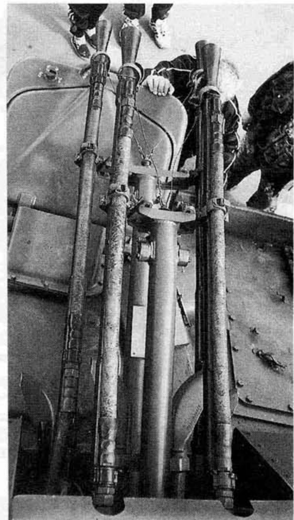
Пушка «Амур». Слева — со сварными трубками отвода охлаждающей жидкости (2А10), справа — с гибкими шлангами (2А10М).
