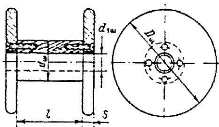
Рисунок 5-2. Конструкция деревянных катушек
