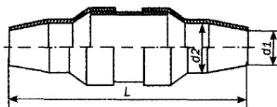
Схема муфты МГНМс 40/66 и 60/77
