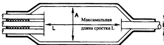
Конструкция муфты XAGA 1000
