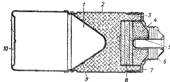
Рис. 15. Корпус гранаты в разрезе:
