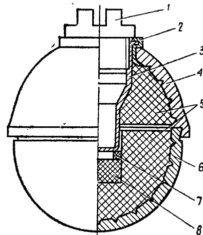
Рис. 11. Устройство ручной гранаты РГН без запала:
