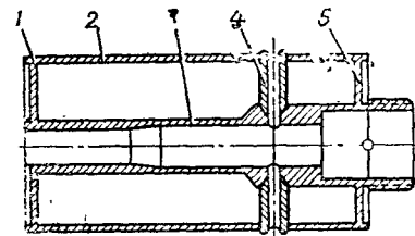
Рис. 39. Корпус гранаты (в разрезе):
