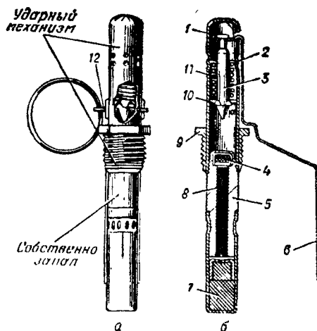
Рис. 4. Запал гранаты УЗРГМ (УЗРГМ-2):
