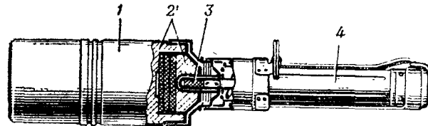
Рис. 14. Устройство ручной противотанковой кумулятивной гранаты РКГ-3:
