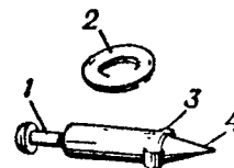
Рис. 5. Ударник и шайба ударника:
