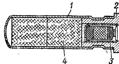
Рис. 19. Запал (в разрезе):
