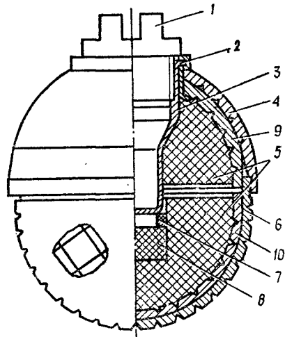
Рис. 12. Устройство ручной гранаты РГО без запала:
