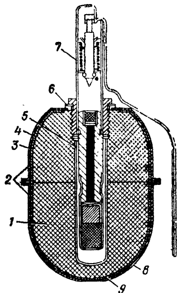
Рис. 3. Устройство ручной осколочной гранаты РГД-5:
