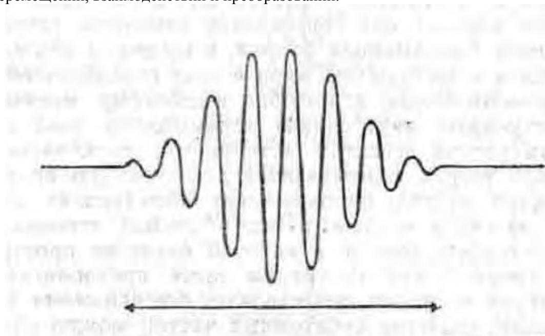
Рис. 27. Сжатие волнового пакета в более малую область
