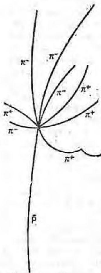
Рис. 37. Возникновение восьми пионов в результате столкновения антипротона и протона
