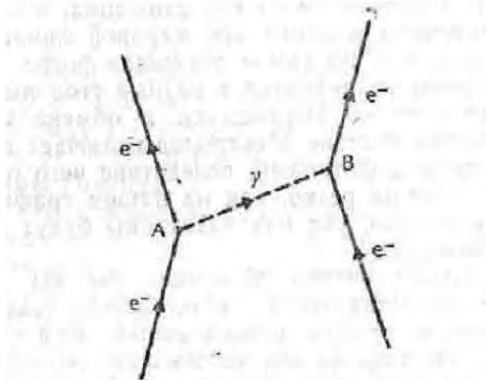
Рис. 29. Взаимное отталкивание двух электронов посредством обмена фотоном
