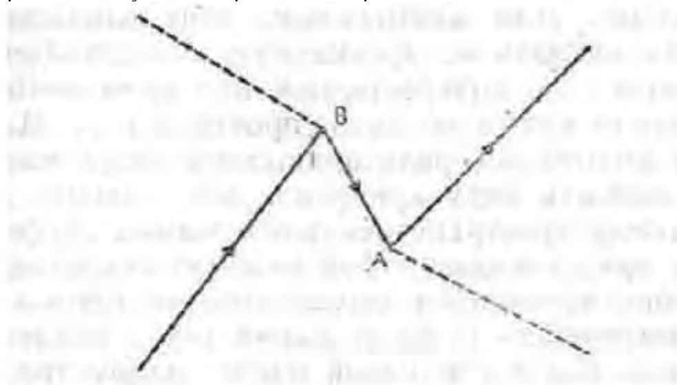
Рис. 25. Процесс рассеивания, включающий фотон, электроны и позитрон.
