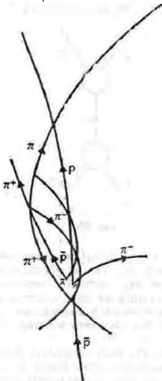
Рис. 55. Сеть реакций, в которых принимают участие протоны, антипротоны, несколько пионов и пара ламбда-антиламбда
