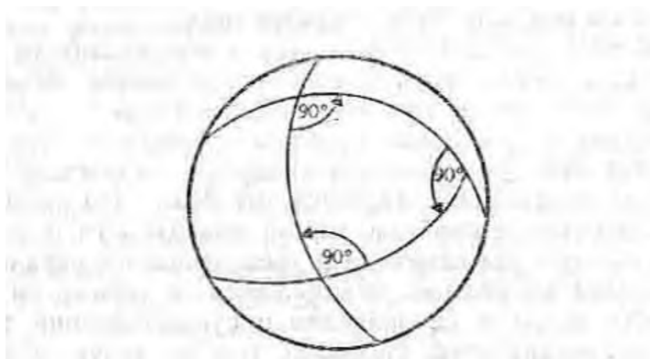
Рис. 18. На сфере треугольник может иметь три прямых угла
