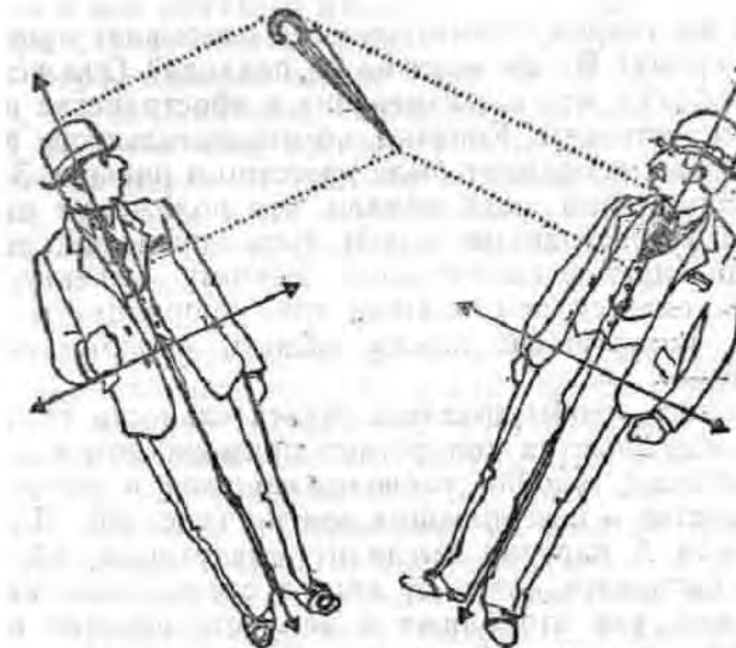
Рис. 16. Два наблюдателя, а и б, рассматривающие зонтик
