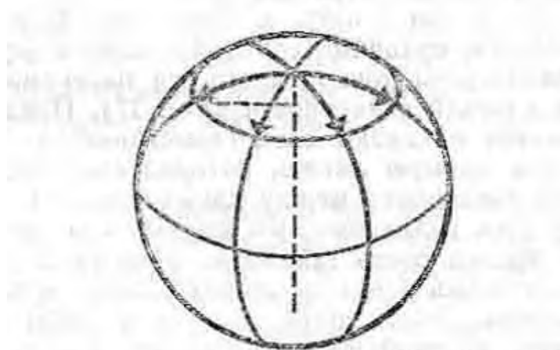
Рис. 19. Начертание круга на сфере
