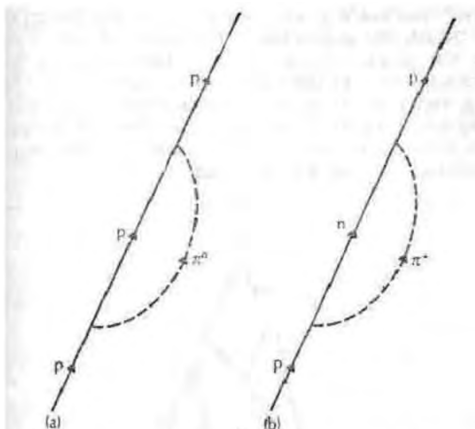
Рис. 42. Фейнмановские диаграммы, показывающие, как протон излучает и поглощает виртуальные пионы
