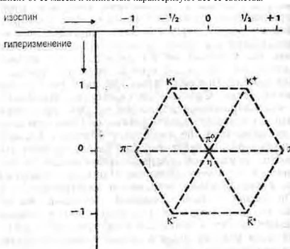
Рис. 48. Мезонный октет
