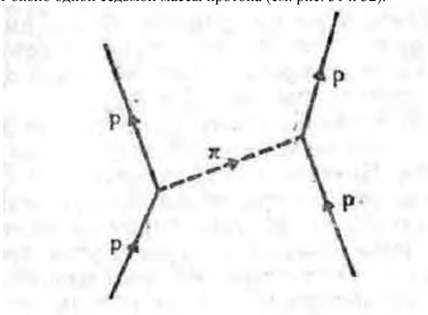
Рис. 31. Два протона обмениваются пионом
