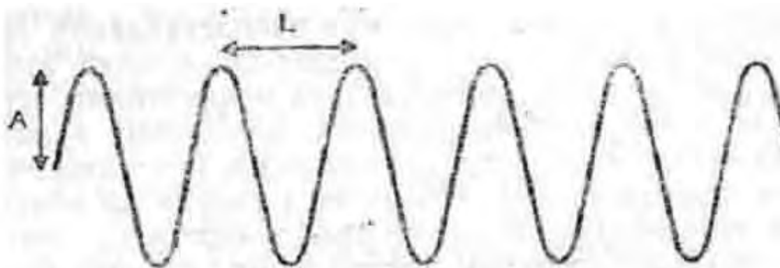
Рис. 14 Волновой паттерн
