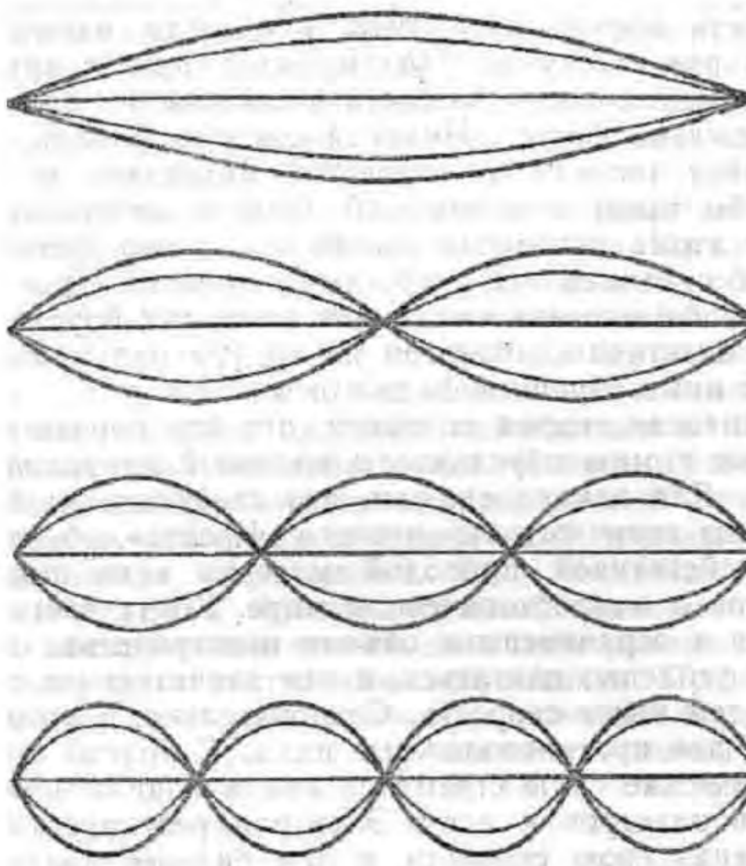
Рис. 6. Стоячие волны в вибрирующей струне
