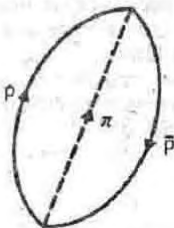
Рис. 33. Вакуумная диаграмм
