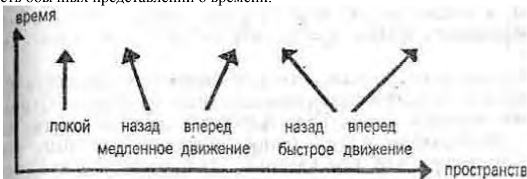
Рис. 20. Мировые линии частиц
