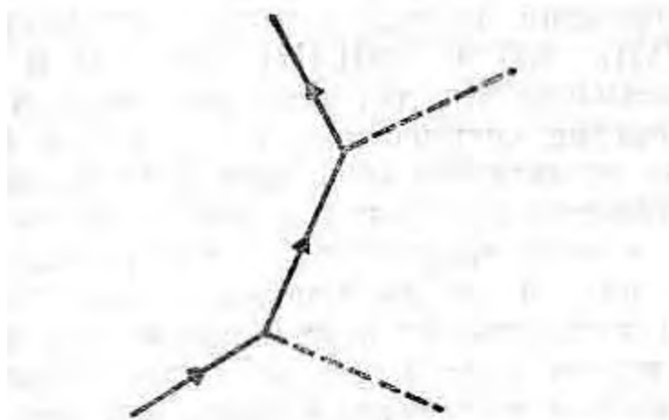
Рис. 22. Электрон-фотонное рассеивание
