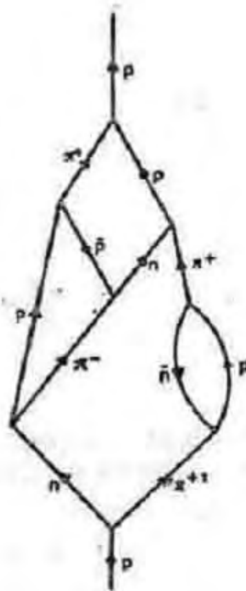
Рис. 44. Сеть виртуальных взаимодействий
