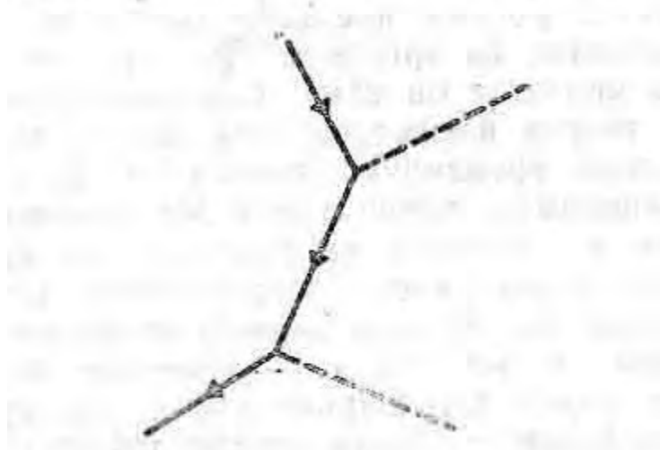
Рис. 23. Позитрон-Фотонное рассивание
