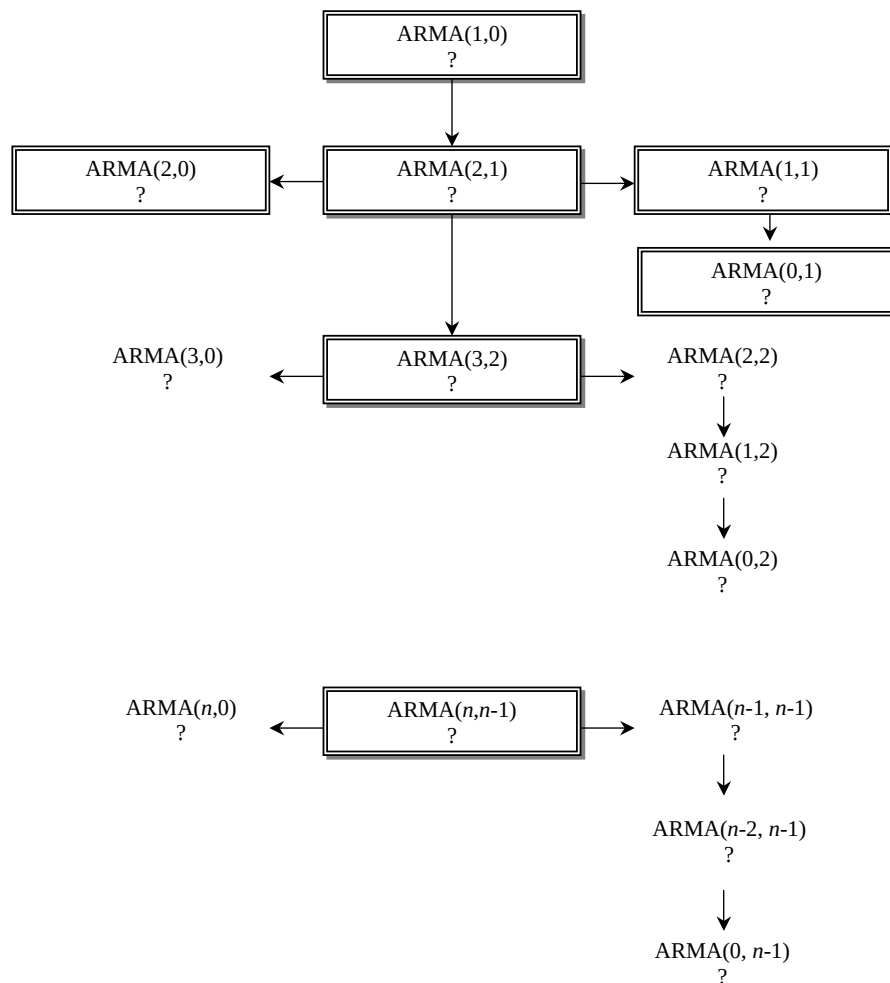
Рис. 15. Процесс выбора ARIMA модели
