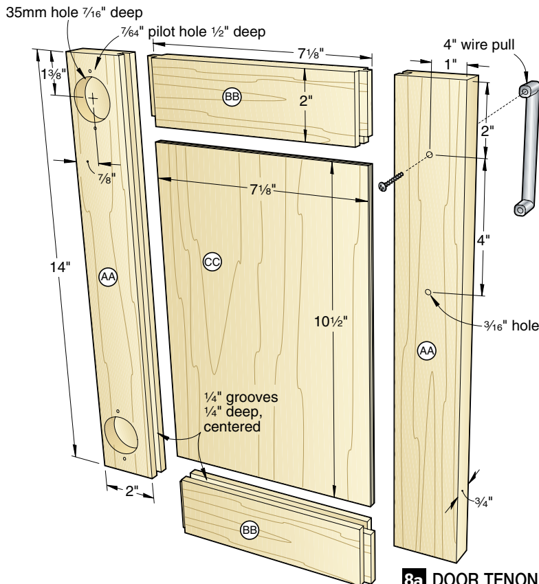
8a DOOR TENON DETAIL
