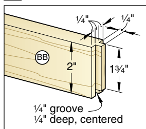
8a DOOR TENON DETAIL
