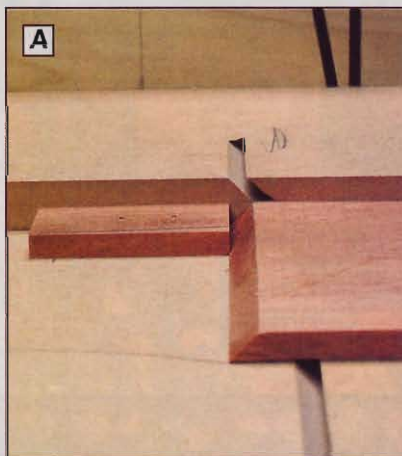
CROSSCUT SLED
