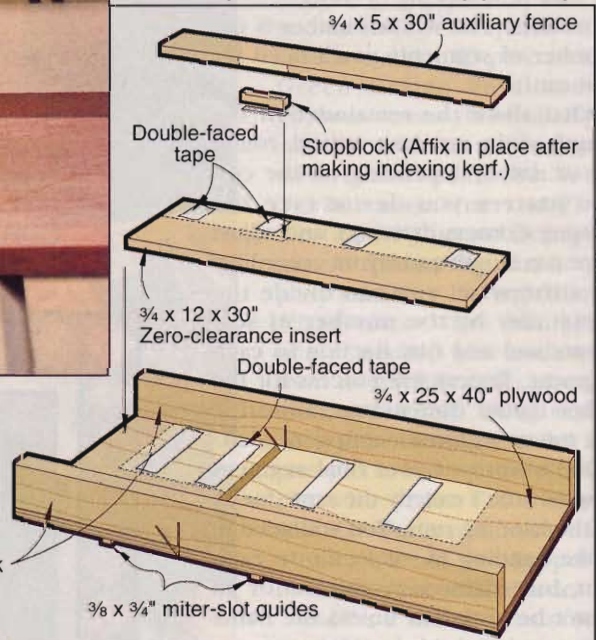
CROSSCUT SLED
