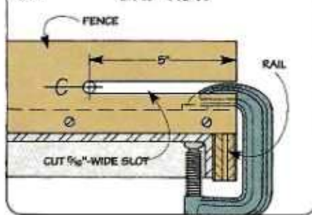
a. END VIEW
