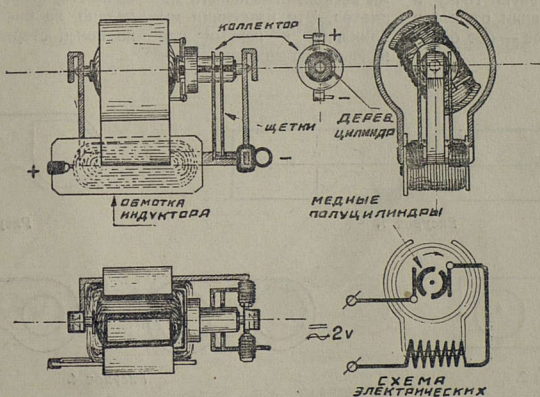
Чертежи и схема соединений электромоторчика.
