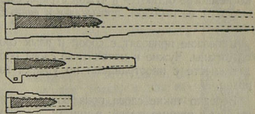
Наверху — ствол пушки, в середине — ствол гаубицы, внизу — ствол-mortиры.
