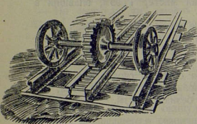
Гребенчатый железный рельс.
