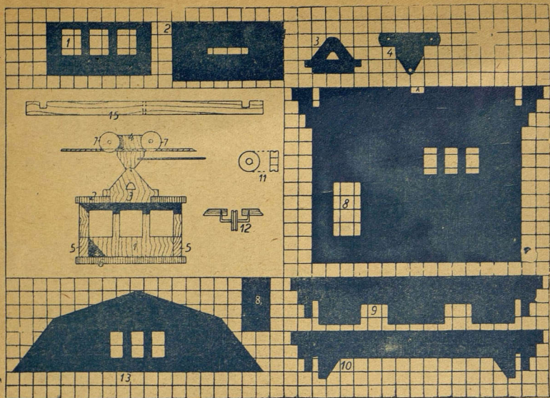
Чертеж вагонетки для подвесной железной дороги.
