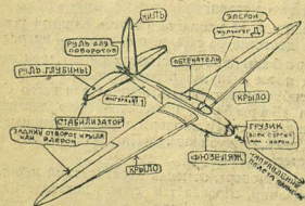
Общий вид модели планера из бумаги
