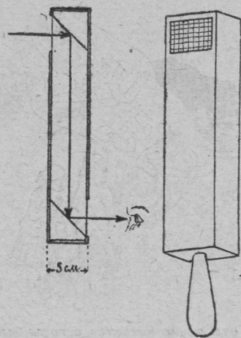
Слева чертёж перископа сбоку; справа общий вид—сверху сетка, чтобы во время игры не разбить зеркало
