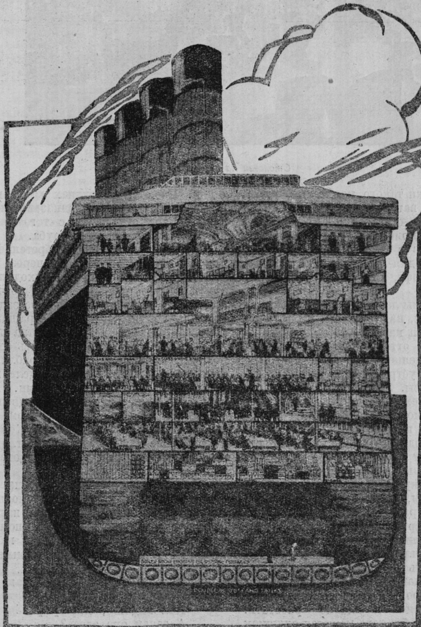
Разрез океанского парохода
