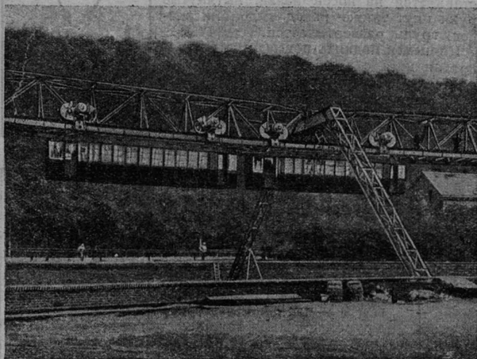
Здесь вагоны находятся не на рельсах, а под рельсами, и поезд катится на тележках, укрепленных над его крышей. Такая железная дорога проведена в Эльдержельде в Германии.
