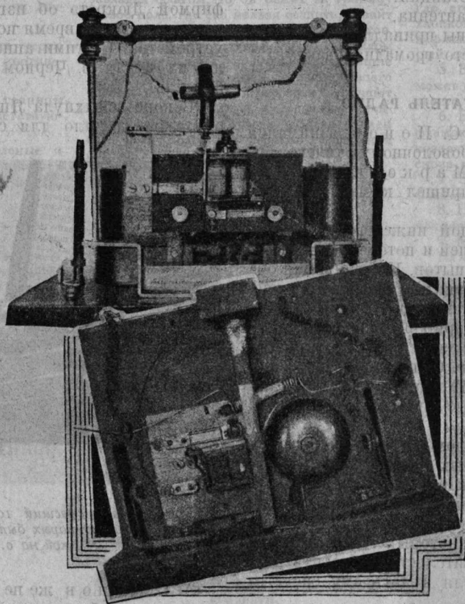
ВВЕРХУ—станция А. С. Попова, сделанная 1889 г. ВНИЗУ—грозоотметчик А. С. Попова 1895 г.
