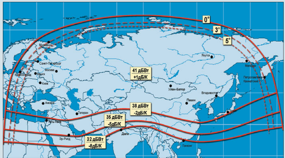
Зона покрытия транспондеров КА «Ямал-100» (90° в.д.)
