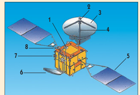
1 – датчик Земли; 2 – антенно-фидерное устройство S-диапазона; 3 – антенна межспутниковой связи; 4 – антенно-фидерное устройство Ka-диапазона; 5 – панель солнечных батарей; 6 – антенна связи с наземной станцией; 7 – электродвигатель постоянного тока; 8 – антенна радиомаяка
