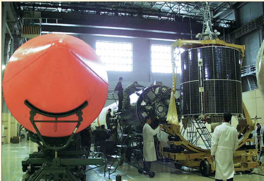
Стыковка космического аппарата с носителем
