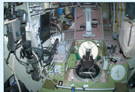
Аппаратура для проведения экспериментов по программе «Релаксация» на борту МКС, установлена на иллюминаторе №9 СМ. Снимок сделан в апреле 2002 г.
