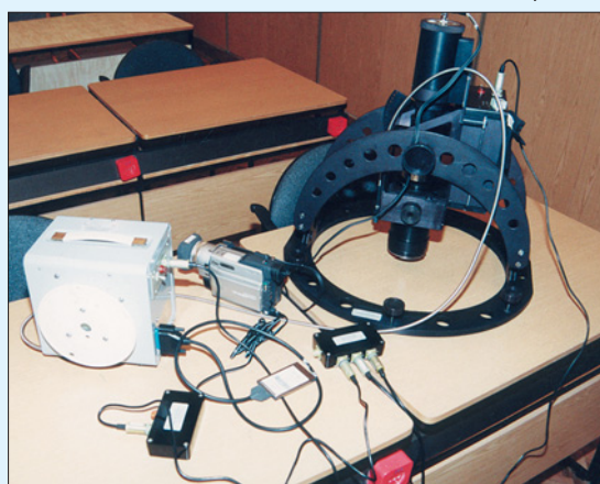
Комплект аппаратуры «Фиалка»
