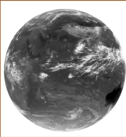
Первые снимки с КА Metsat-1, полученные 19–20 сентября в трех спектральных диапазонах – тепловом ИК (TIR), видимом (VIS) и в линии водяного пара (WVIR)
