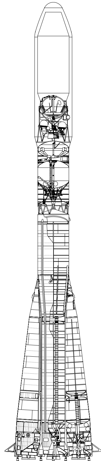
Схема ракетно-космического комплекса «Аврора»
