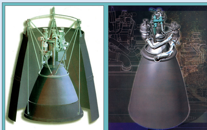
Для удешевления разработки (и не только) американцы стремятся разрабатывать двигатели нового поколения вместе с европейцами (SPW2000, ранее известен как RL50, фото слева) или с японцами (MB60, справа).
