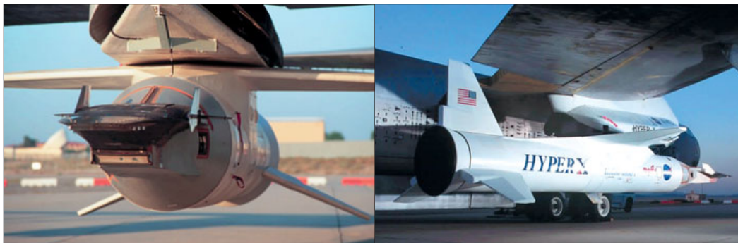
Перед штурмом гиперзвука. Нурег-Х на пилоне под крылом В-52 – вид спереди (слева) и сзади
