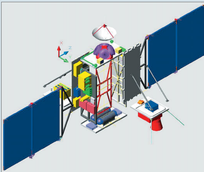
Конструктивно-технологическое членение МКА Д33, на базе которого будут создаваться КА проекта ЕМЕС. Рисунок КБ «Полет»
