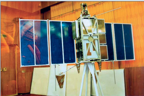
Макет платформы МКА Д33, на базе которой планируется создавать КА проекта ЕМЕС. Фото КБ «Полюс»
