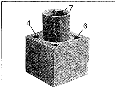
Элемент жаропрочного керамического двигателя.
