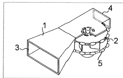
Ветроэнергетический преобразователь.
