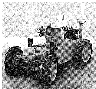
Робототехнический комплекс радиационной разведки.
