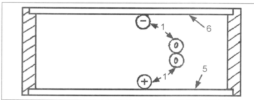
Рис. 3. Сосуд с вакуумом.
