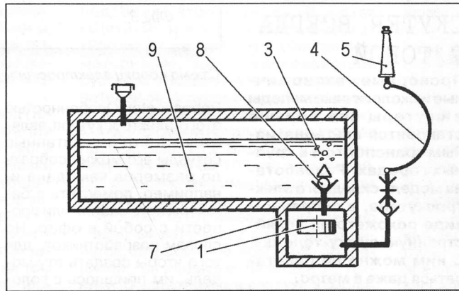
Рис.1. Установка пожаротушения. Общий вид.
