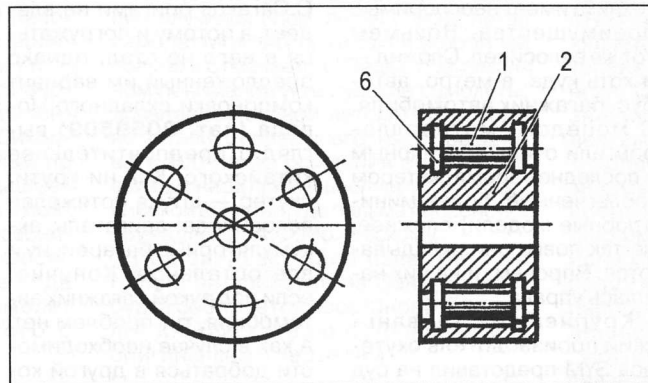
Рис.2. Барабан зарядов.
