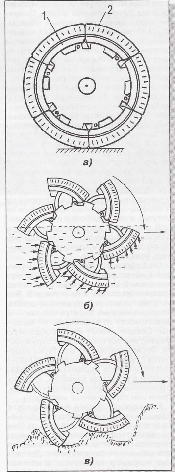
Новый движитель, способный преодолевать любое бездорожье: в колесном варианте на асфальте (а), движется по воде (б), пересеченной местности (в).
