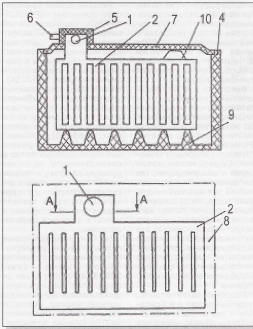
Схемы батареи.
