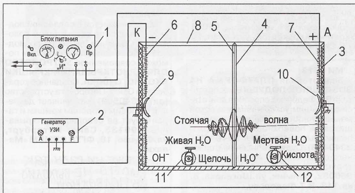
Схема промышленной установки электроактивации воды: 1) блок питания; 2) генератор УЗИ; 3) корпус; 4) рамка диафрагмы; 5) диафрагма из целлофана или пористой керамики; 6) катод из активированного наногуглерода; 7) анод из активированного наногуглерода; 8) крышка корпуса; 9—10) пьезоэлементы УЗИ; 11) кран живой воды; 12) кран мертвой воды.
