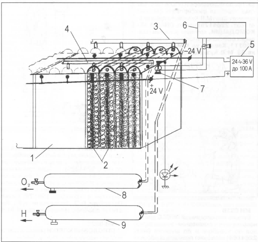
1) корпус аккумулятора 6СТ-60, 2) пластины УВС, 3) газовый коллектор водорода, 4) газовый коллектор кислорода, 5) источник постоянного тока, 6) бак водного раствора КОН на 10 л, 7) поплавок с клапаном уровня жидкости, 8) ресивер кислорода на 10 л, 9) ресивер водорода на 15 л.
