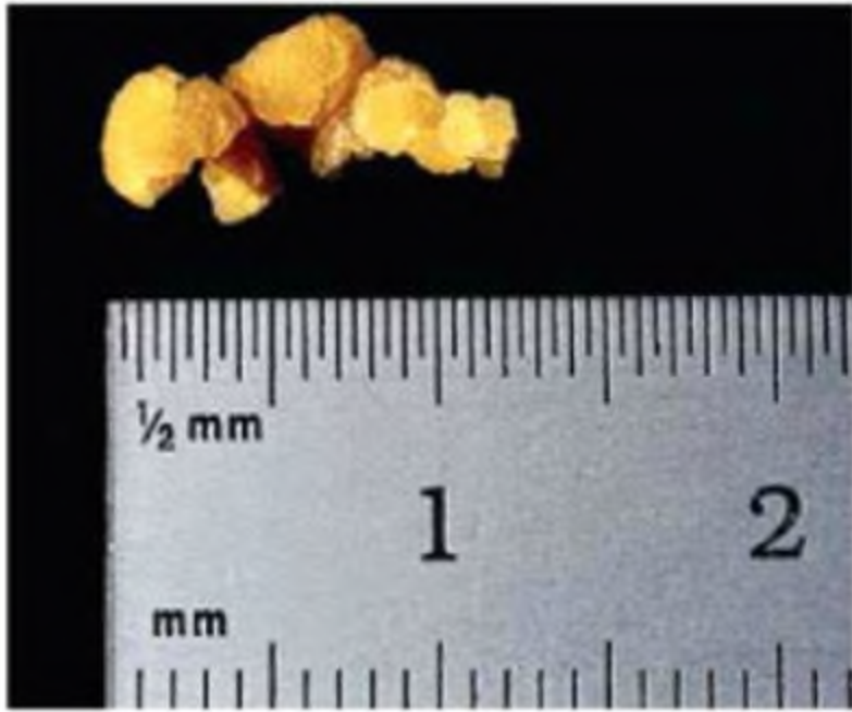
Размер кусочков кальцита, найденных в альпийских ледяных пещерах и изучаемых в лаборатории Инсбрукского университета, — всего несколько миллиметров. Но они хранят массу ценной информации об истории Земли
