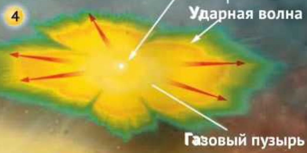
Нейтронная звезда
