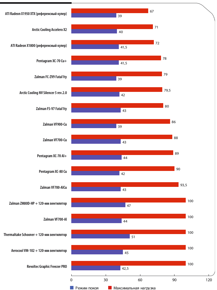
Температура ядра Radeon X1950 XTX, °C
