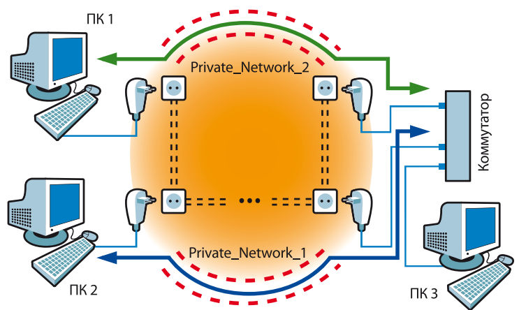
Тестовая ситуация: две виртуальные подсети образованы на одной и той же паре проводов питающей проводки
